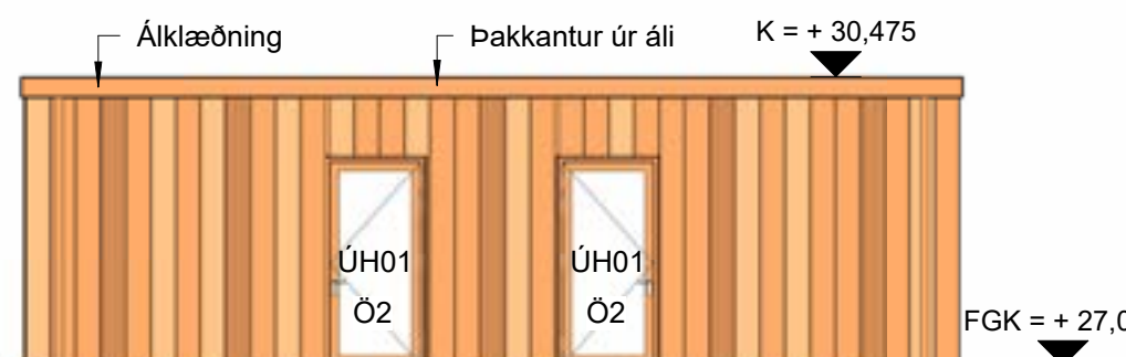
Ásýnd 1 - Geymsluskúr
