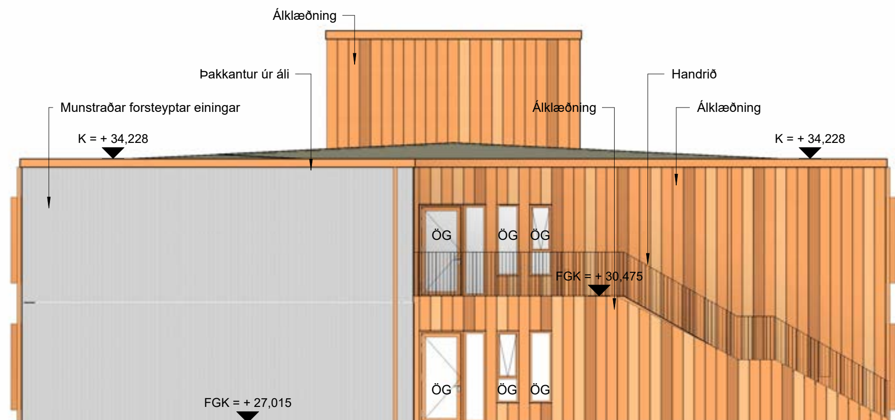
Ásýnd 7 - a Suður mkv: 1 : 100
