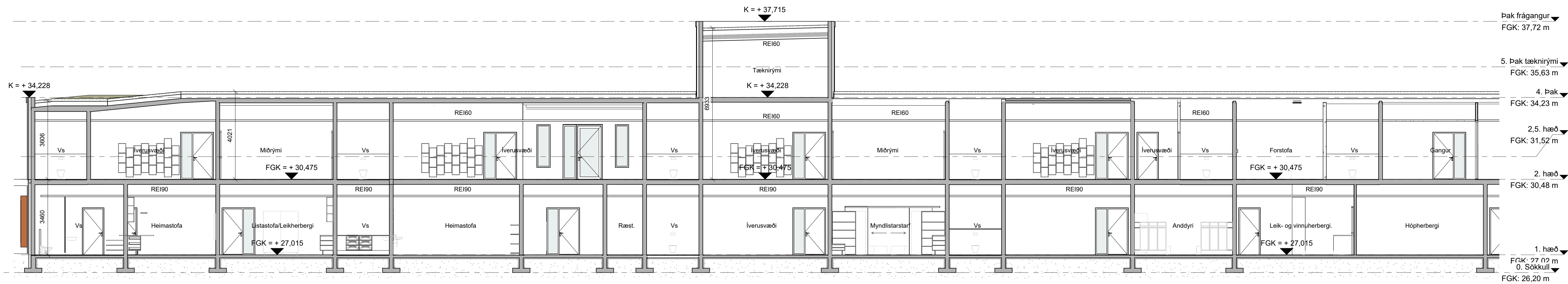
F mkv: 1 : 100
