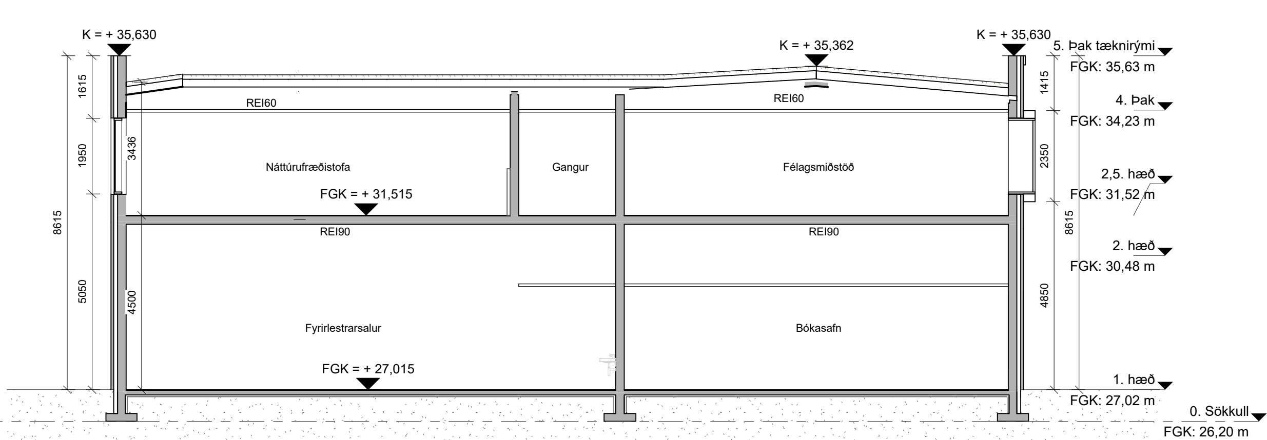
2 mkv: 1 : 100
