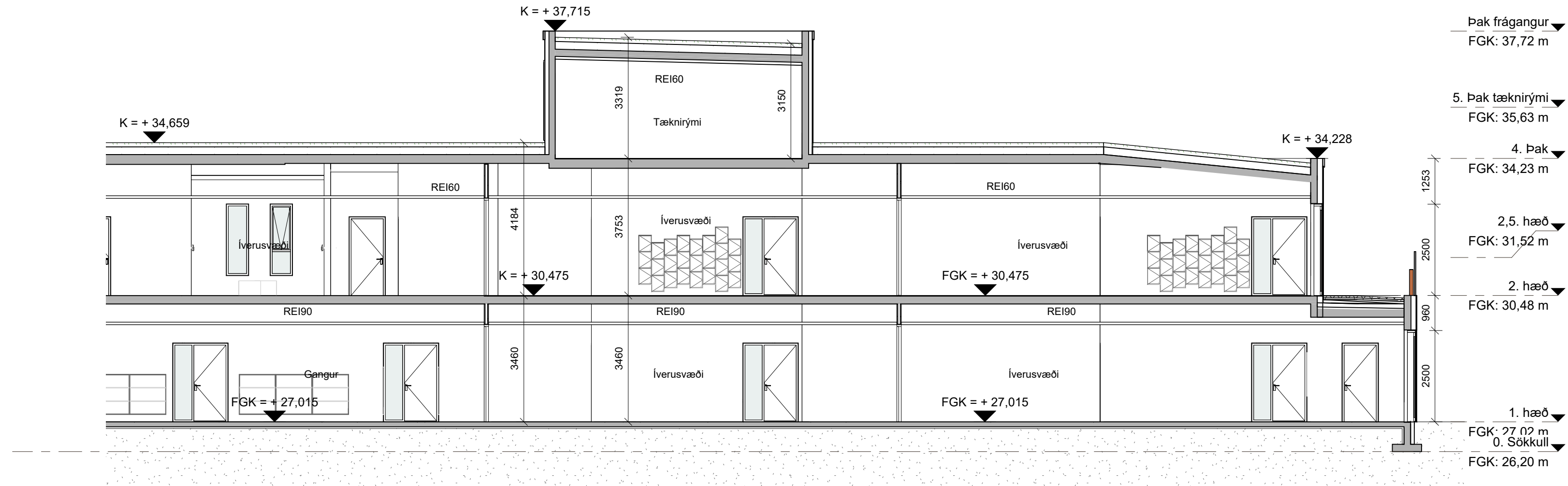
H mkv: 1 : 100
